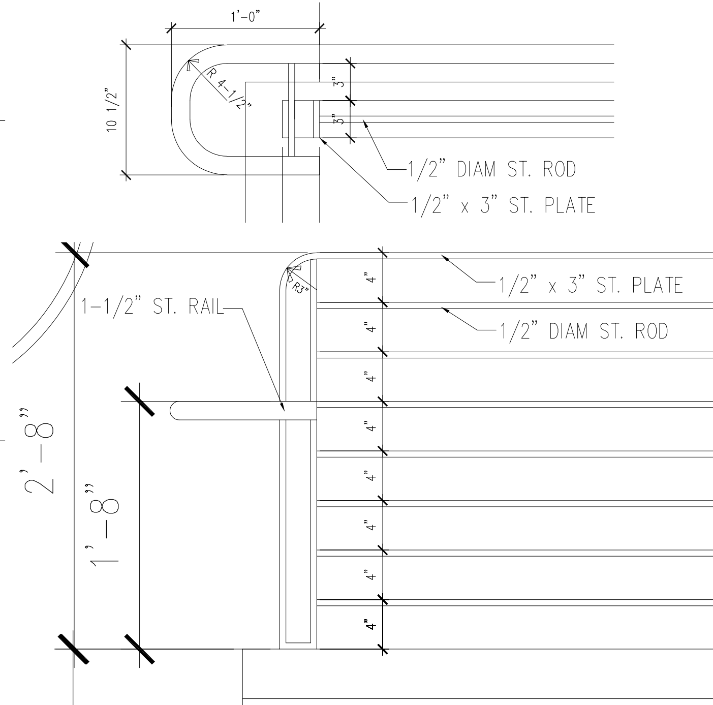
8 RAILING DETAIL A-300 SCALE: 1-1/2" = 1'-0"
