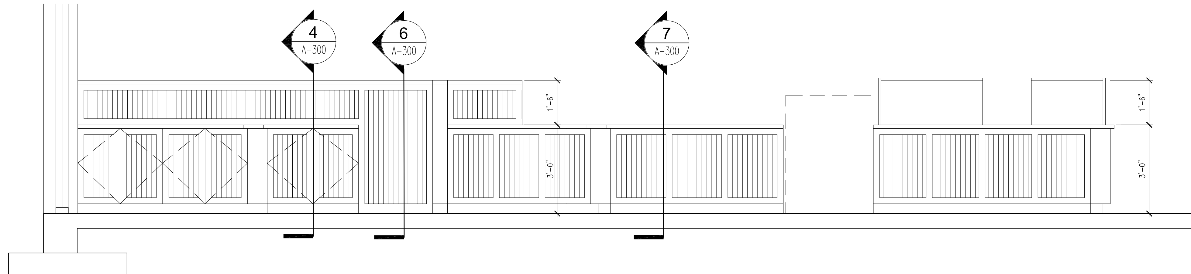
2 CASEWORK ELEVATION A-300 SCALE: 1/2" = 1'-0"
