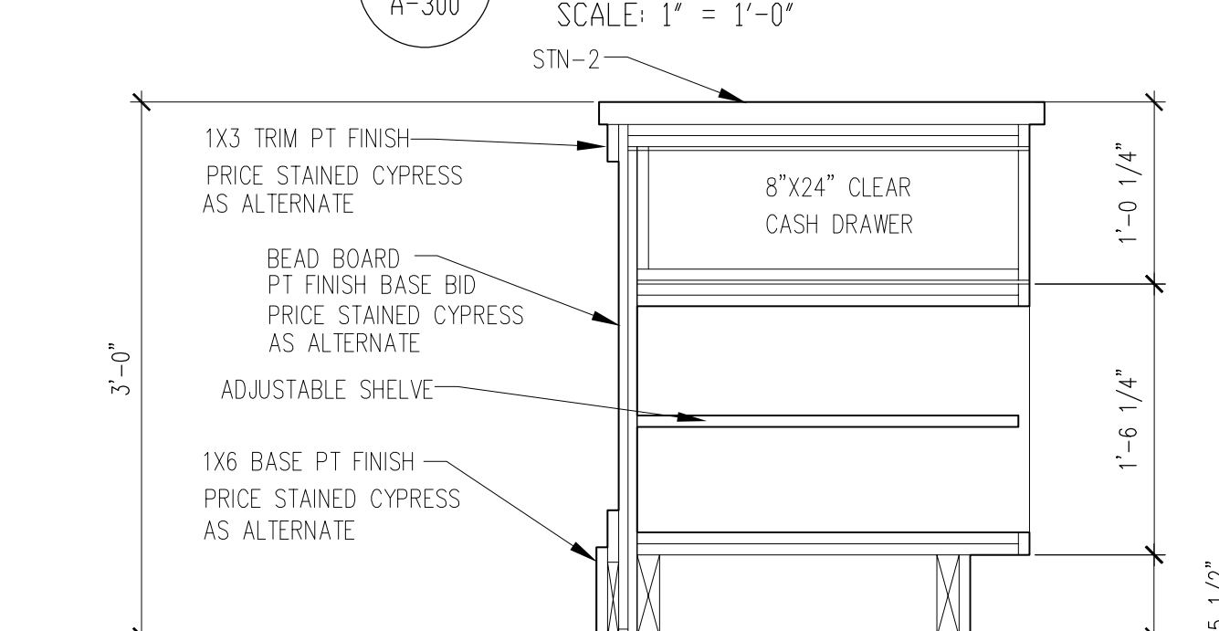
7 CASEWORK SECTION A-300 SCALE: 1" = 1'-0"
