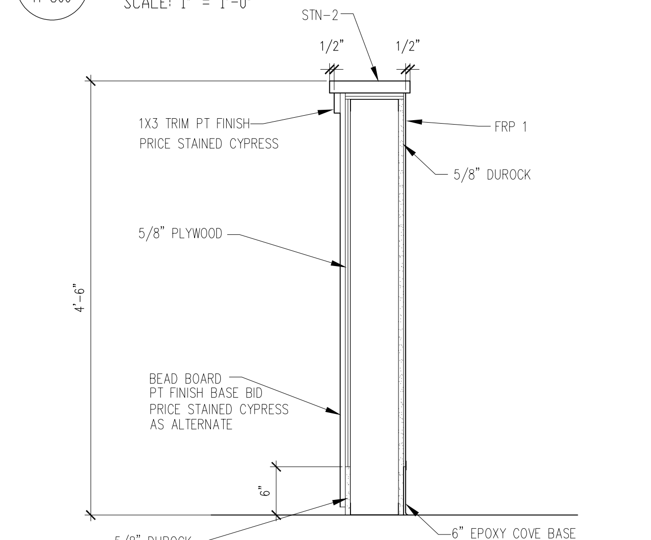
6 CASEWORK SECTION A-300 SCALE: 1" = 1'-0"
