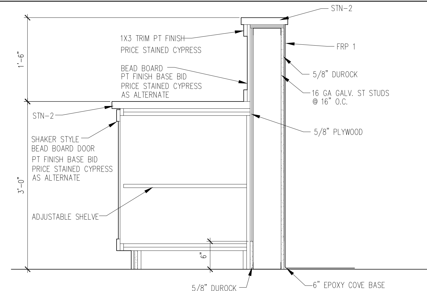
4 CASEWORK SECTION A-300 SCALE: 1" = 1'-0"
