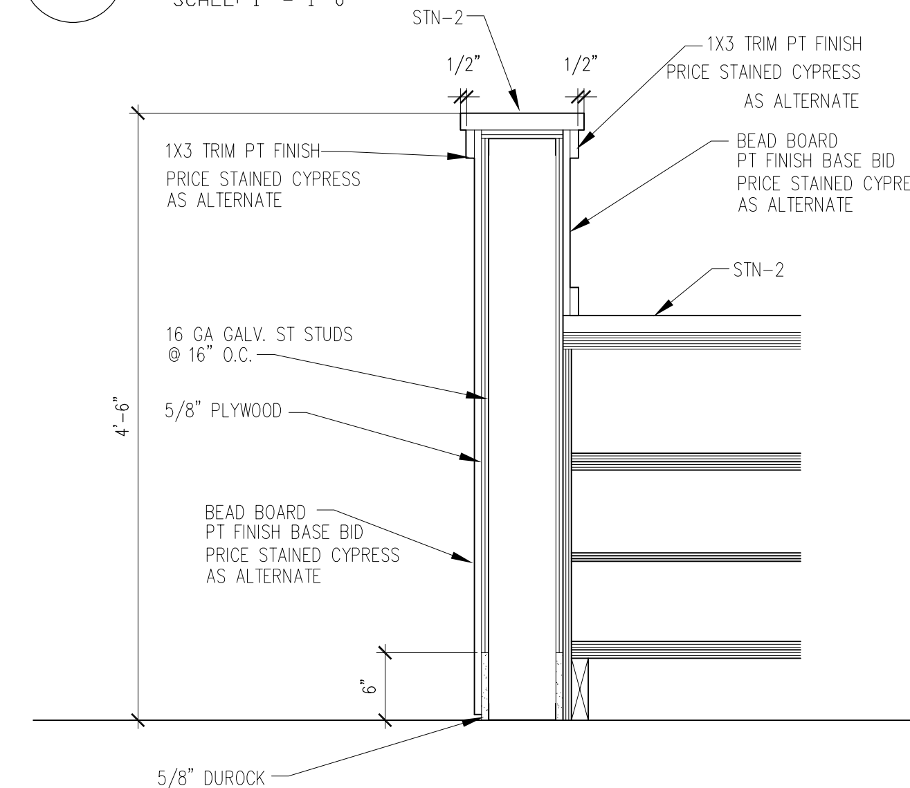
5 CASEWORK SECTION A-300 SCALE: 1" = 1'-0"
